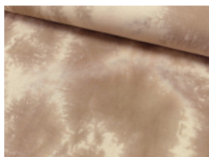
A287K
